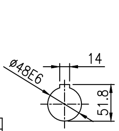
INPUT KEY
