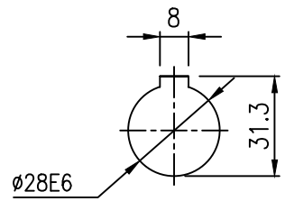
INPUT KEY
