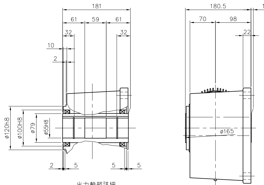
出力軸部詳細
