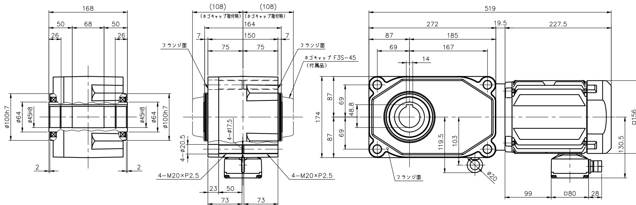
出力軸部詳細
