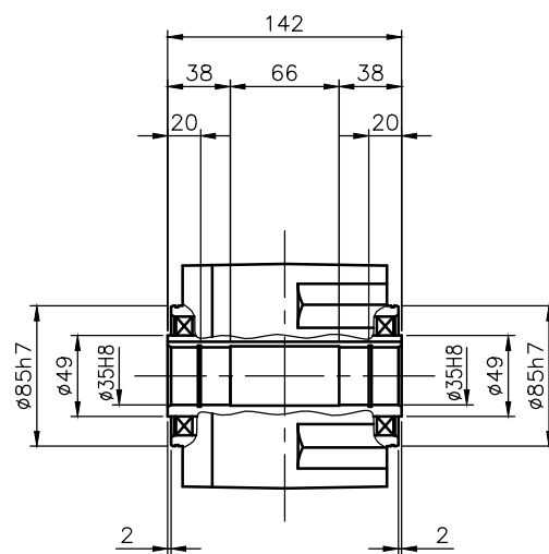
出力軸部詳細
