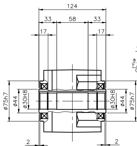
出力軸部詳細
