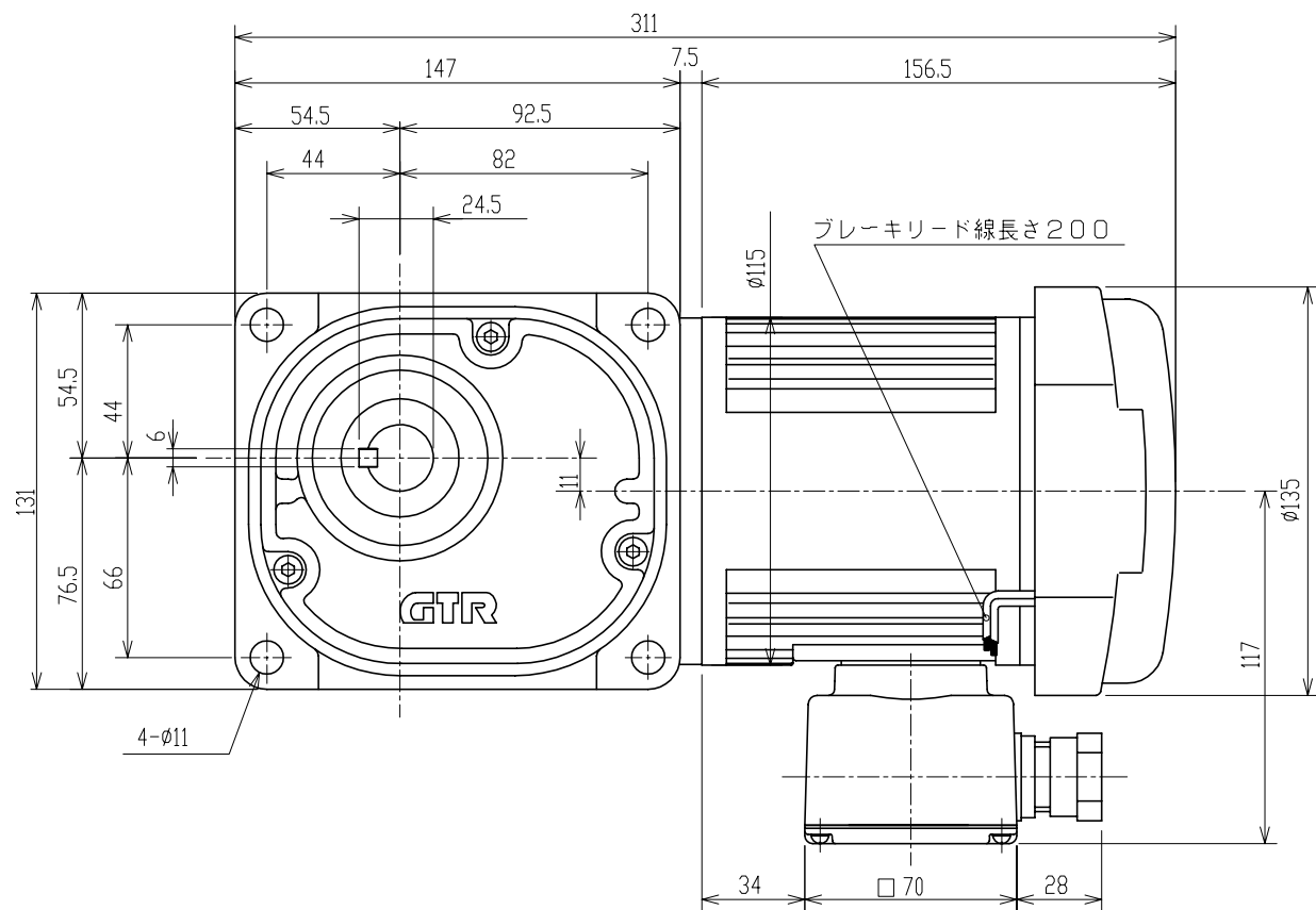
減速機仕様
