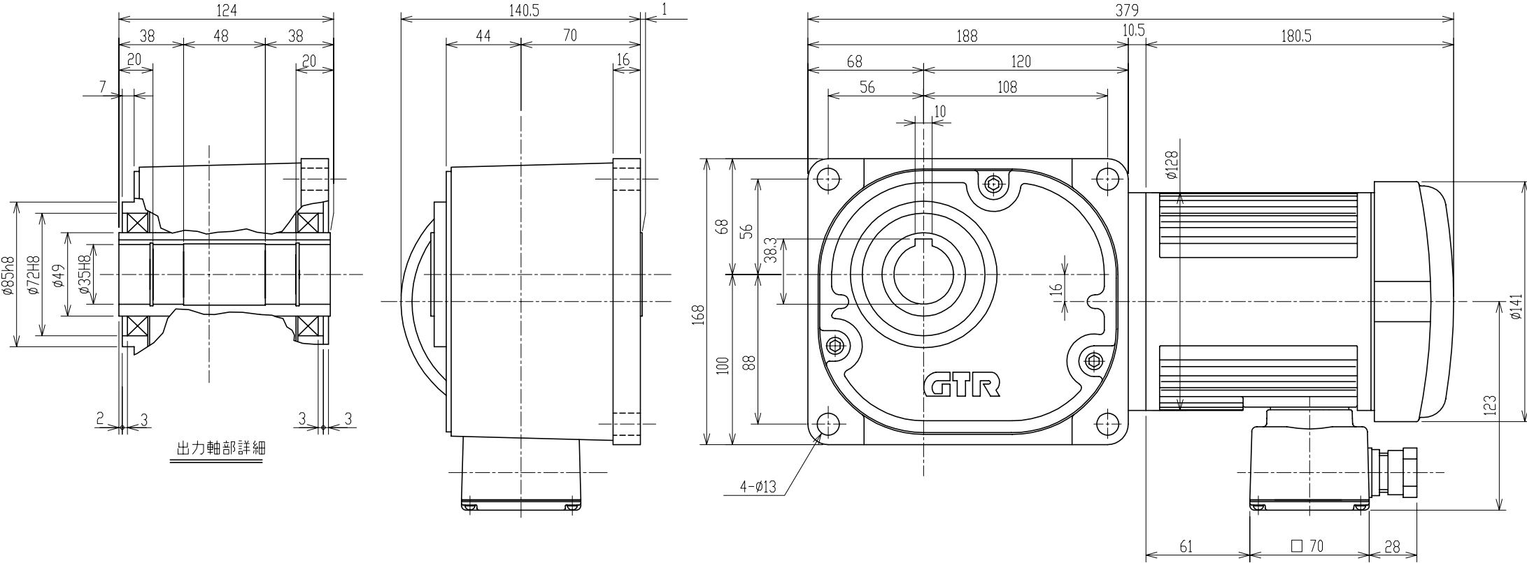
モータ仕様
