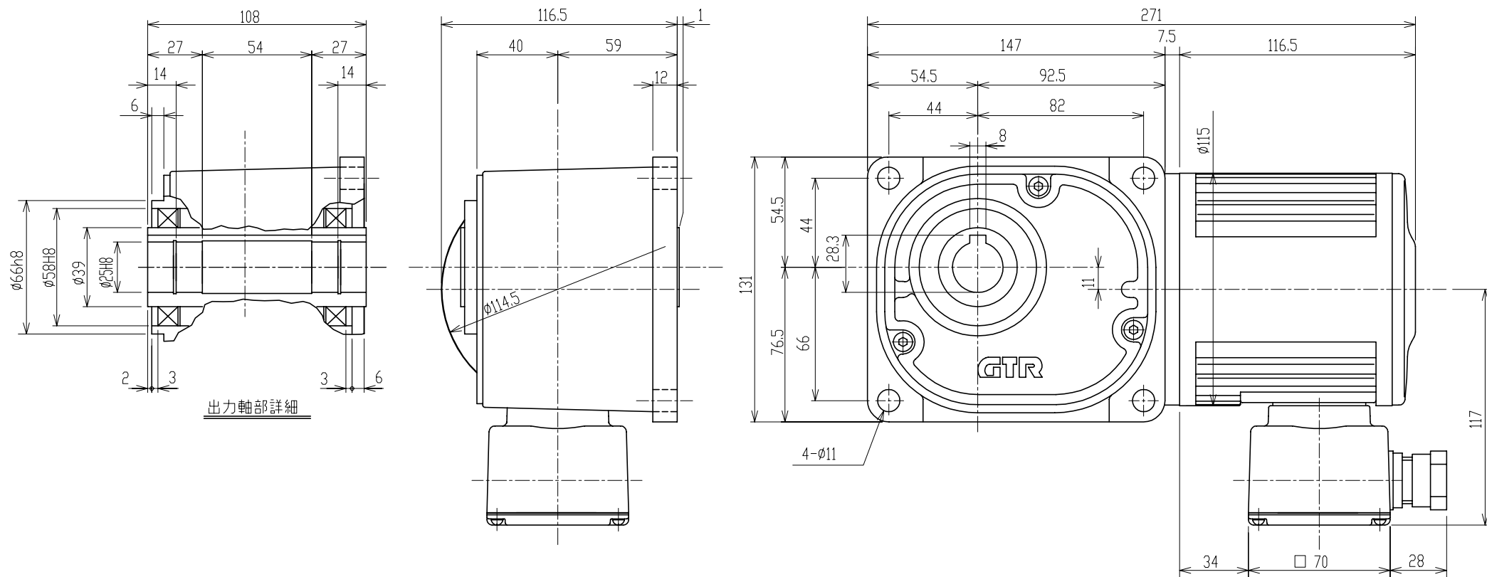
モータ仕様
