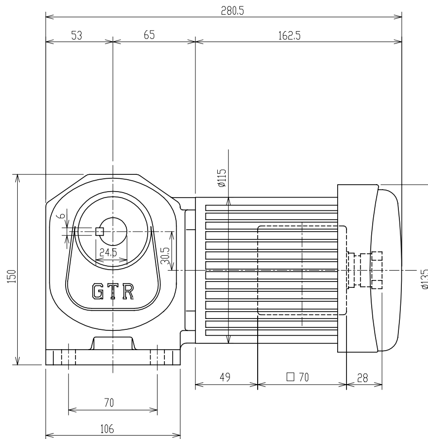
減速機仕様
