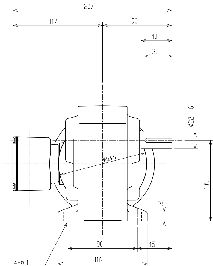
モータ仕様
