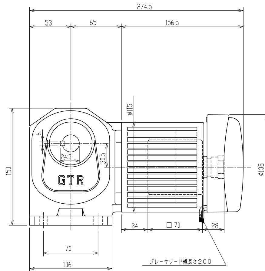
減速機仕様
