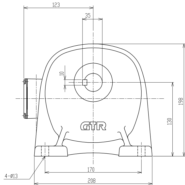
減速機仕様
