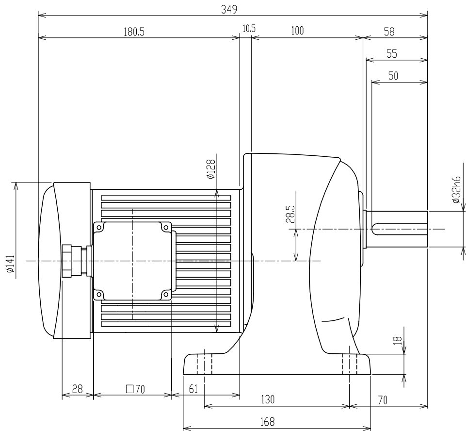
モータ仕様
