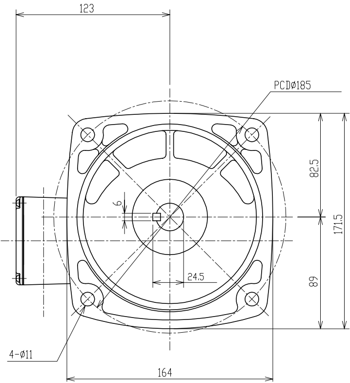
減速機仕様
