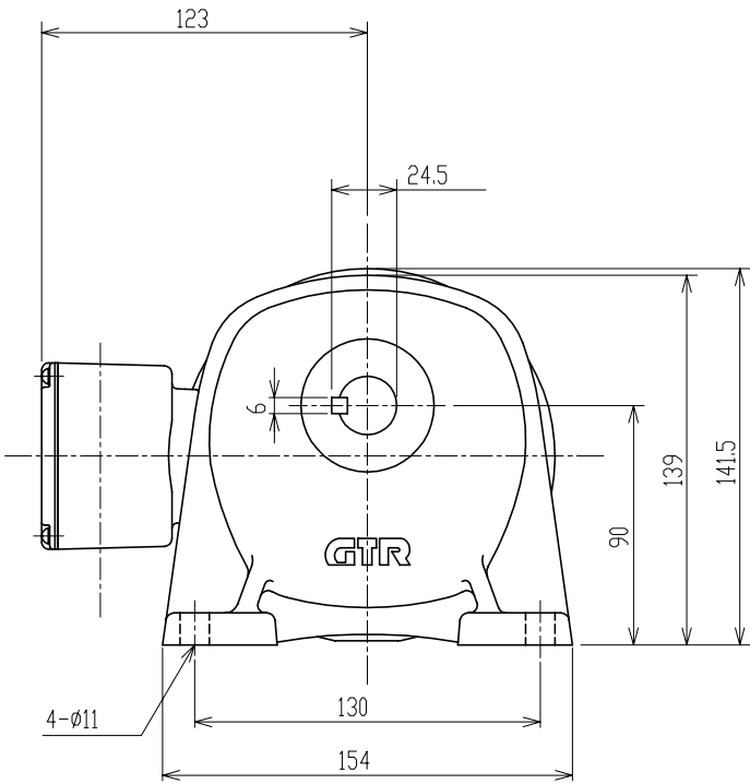
減速機仕様
