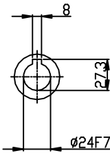
INPUT SHAFT
