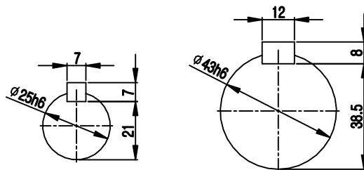
INPUT SHAFT
