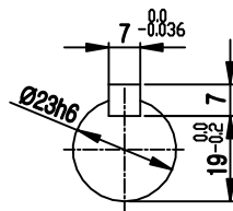
INPUT SHAFT
