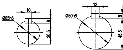
INPUT SHAFT
