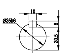
INPUT SHAFT
