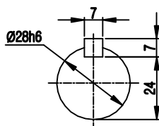
INPUT SHAFT
