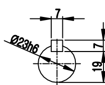
INPUT SHAFT
