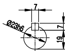
INPUT SHAFT
