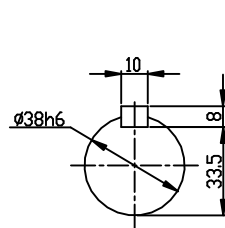
INPUT SHAFT
