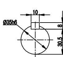
INPUT SHAFT
