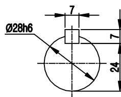
INPUT SHAFT
