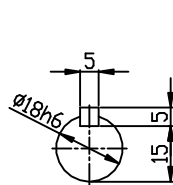
INPUT SHAFT
