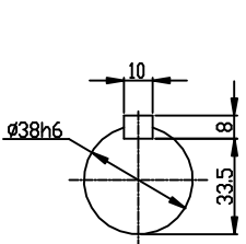
INPUT SHAFT
