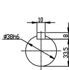
INPUT SHAFT
