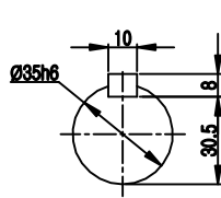
INPUT SHAFT
