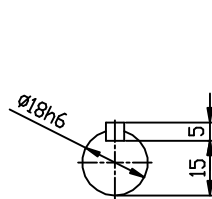
INPUT SHAFT
