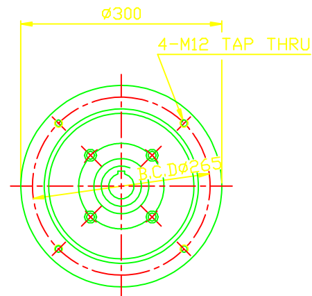
MOTOR FLANGE
