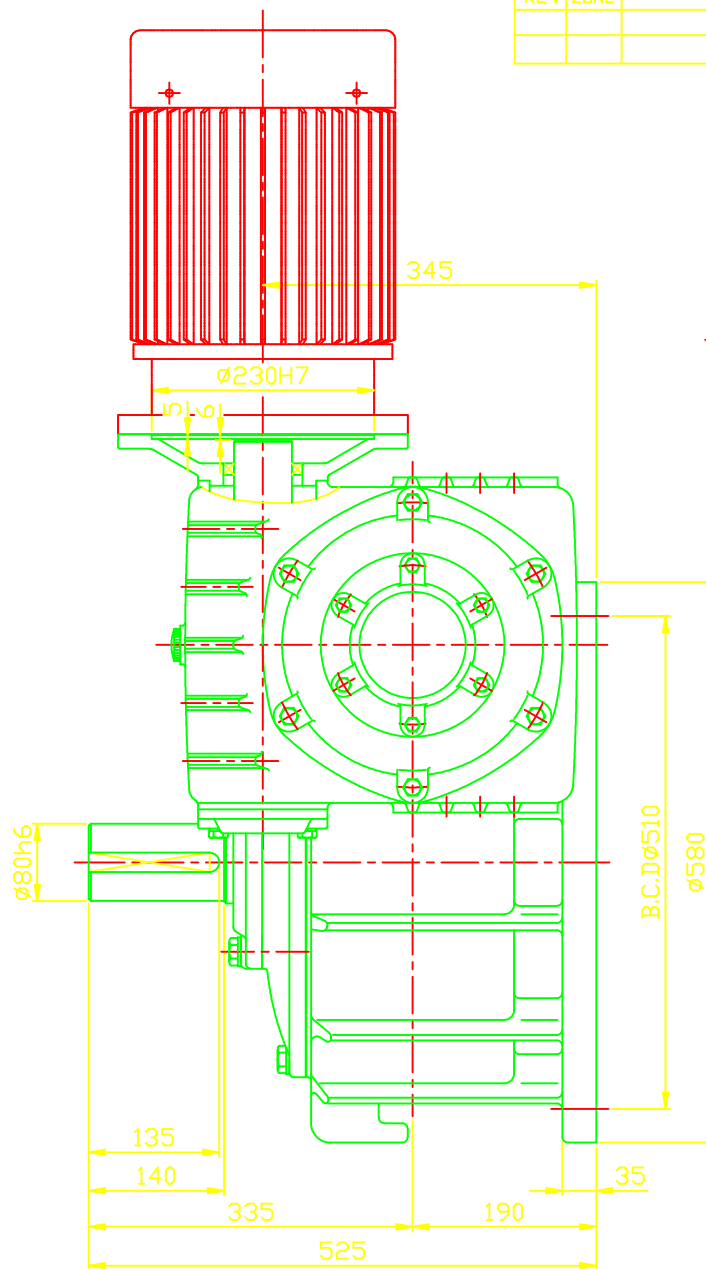
MOTOR FLANGE
