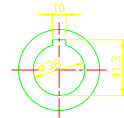
INPUT SHAFT
