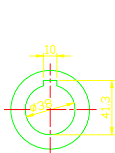
INPUT SHAFT
