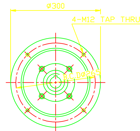
MOTOR FLANGE
