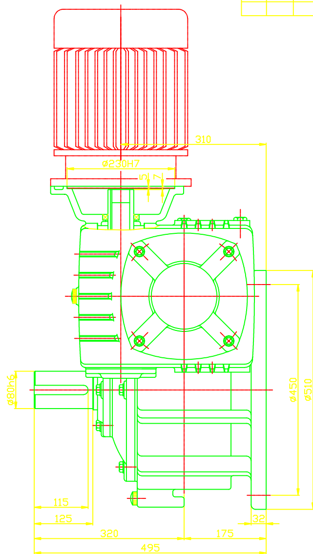
INPUT SHAFT
