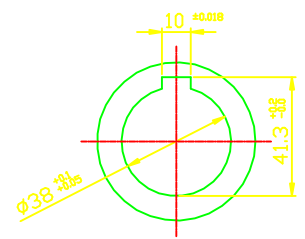
INPUT SHAFT
