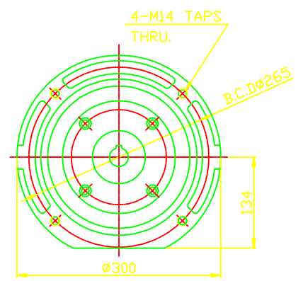
INPUT SHAFT
