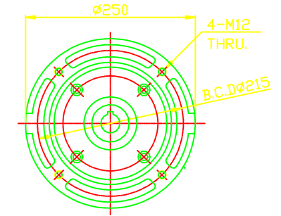
INPUT SHAFT
