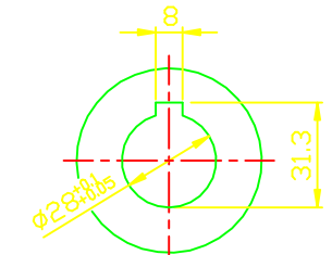
INPUT SHAFT
