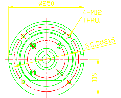
MOTOR FLANGE
