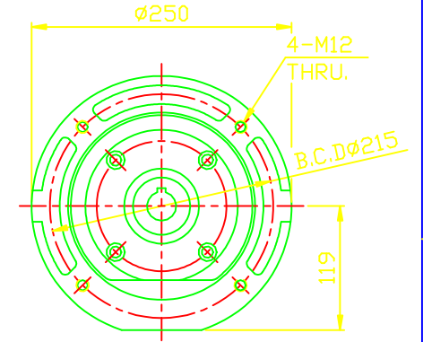
MOTOR FLANGE
