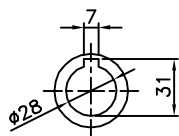
INPUT SHAFT
