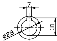
INPUT SHAFT
