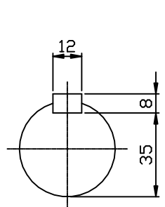
INPUT SHAFT
