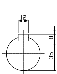
INPUT SHAFT
