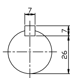
INPUT SHAFT
