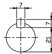
INPUT SHAFT
