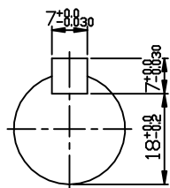
INPUT SHAFT
