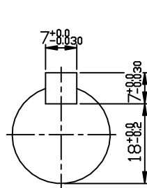
INPUT SHAFT
