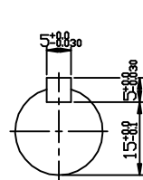
INPUT SHAFT
