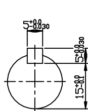
INPUT SHAFT
