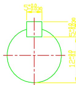
INPUT SHAFT
