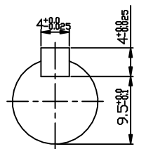
INPUT SHAFT
